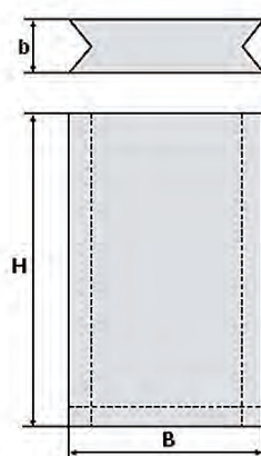
Figur 2 Pinchbotten med invikta sidor alt rak botten utan invikta sidor. I tabellerna anges måtten på produkterna med invikta sidor som B/b x H. Produkter utan invikta sidor anges som B x H
