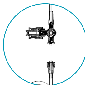
Produkter med 3-vägskran och injektionsmembran: REF 10582-01
