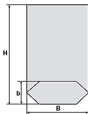
Figur 1 Kanisterbotten
