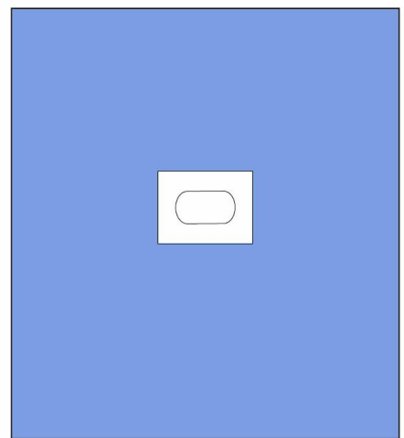
120 x 150 cm ø 5 x 7 cm
