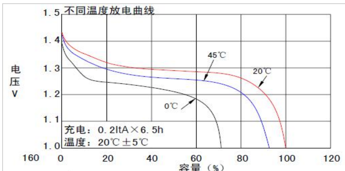
特征曲线
