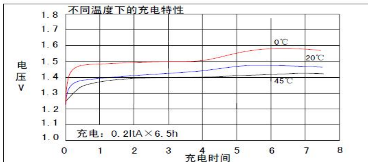
特征曲线
